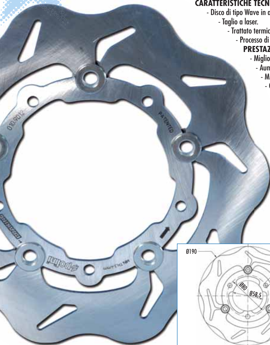
175.0001 spessore / thickness 4 mm.
