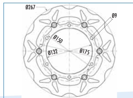
175.0008 spessore / thickness 5 mm.
