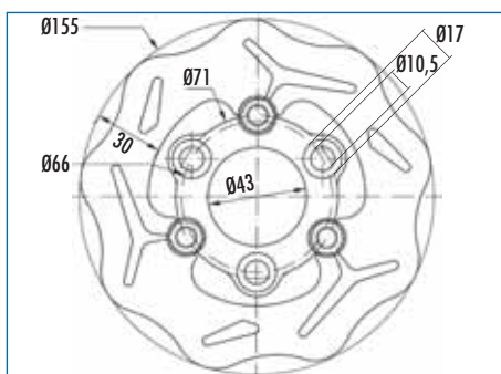
175.0004 spessore / thickness 4 mm.
