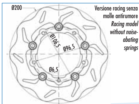
175.0007 spessore / thickness 4 mm.
