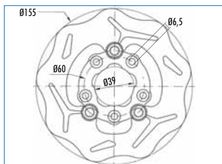
175.0003 spessore / thickness 4 mm.
