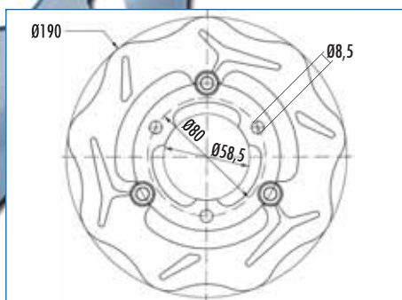
175.0001 spessore / thickness 4 mm.
