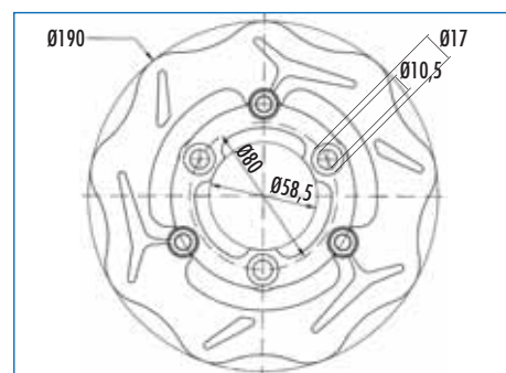
175.0005 spessore / thickness 4 mm.
