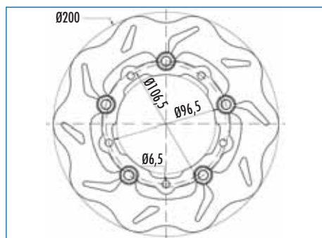
175.0006 spessore / thickness 4 mm.
