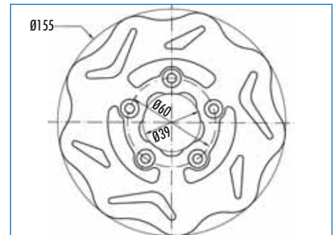
175.0013 spessore/thickness 4 mm.
