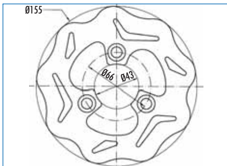
175.0014 spessore/thickness 4 mm.
