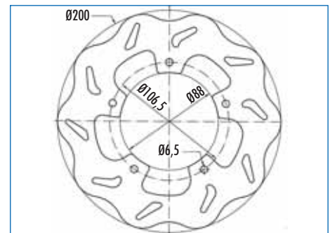
175.0016 spessore/thickness 4 mm.
