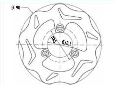
175.0015 spessore/thickness 4 mm.
