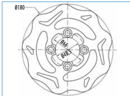
175.0012 spessore/thickness 4 mm.
