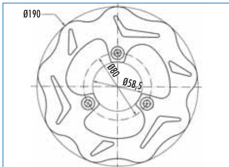
175.0011 spessore/thickness 4 mm.
