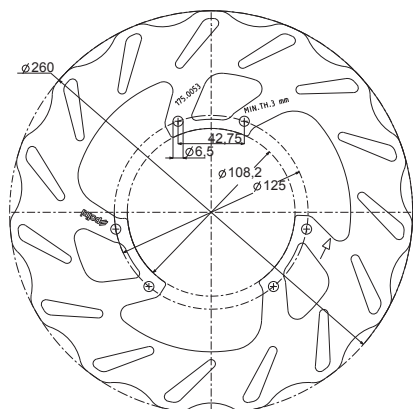
175.0053 thickness/spessore 3,5 mm.
