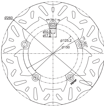
175.0037 thickness/spessore 5 mm.
