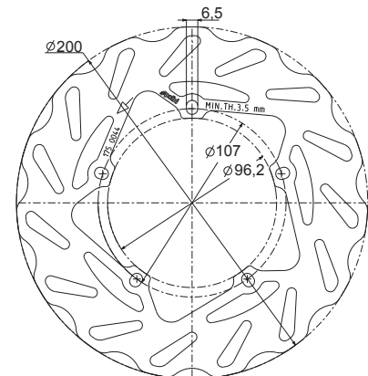
175.0044 thickness/spessore 4 mm.
