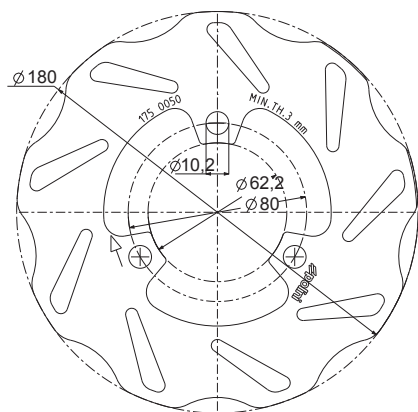
175.0050 thickness/spessore 3,5 mm.
