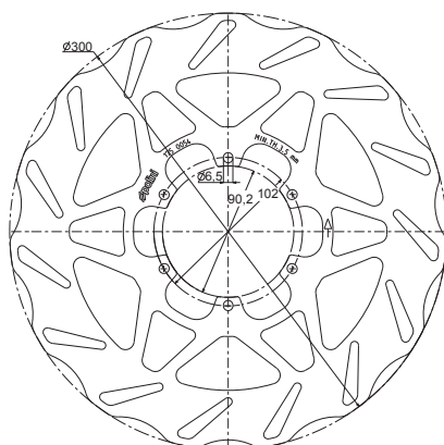
175.0054 thickness/spessore 4 mm.
