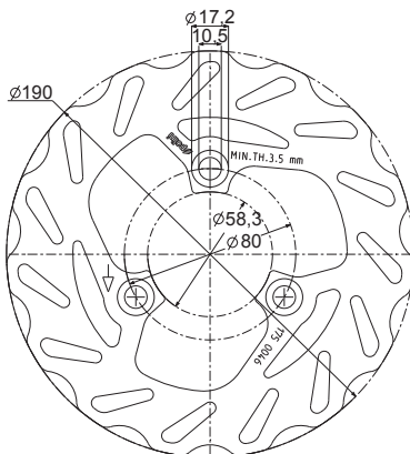
175.0046 thickness/spessore 4 mm.
