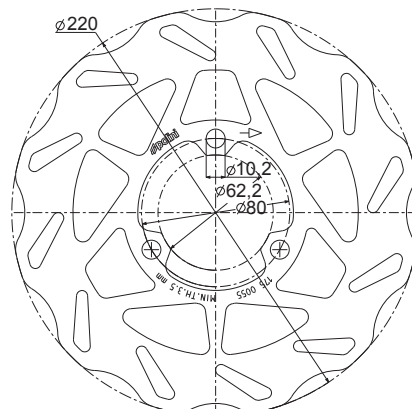
175.0055 thickness/spessore 4 mm.
