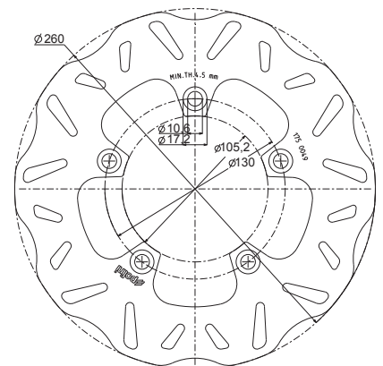
175.0049 thickness/spessore 5 mm.
