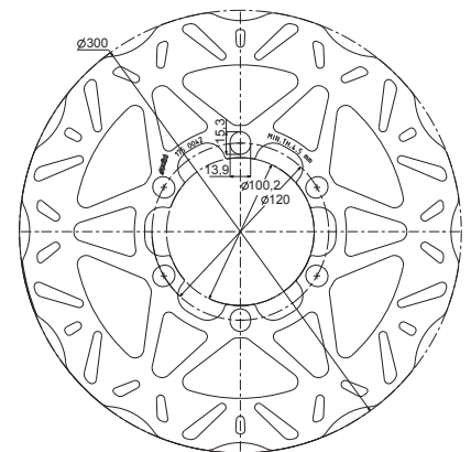
175.0042 thickness/spessore 5 mm.
