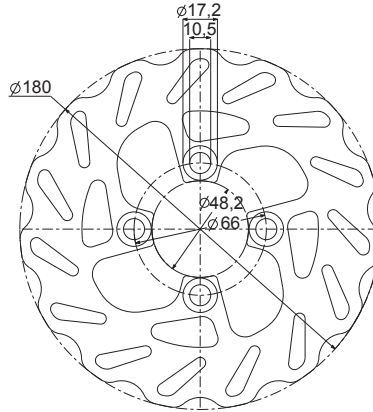
175.0038 thickness/spessore 3,5 mm.
