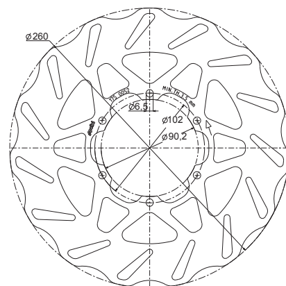
175.0052 thickness/spessore 4 mm.
