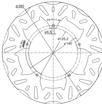
175.0041 thickness/spessore 4 mm.
