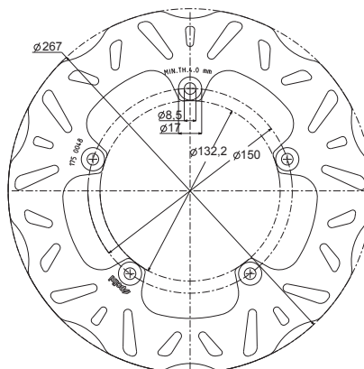
175.0048 thickness/spessore 4,5 mm.
