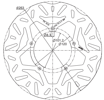
175.0039 thickness/spessore 5 mm.
