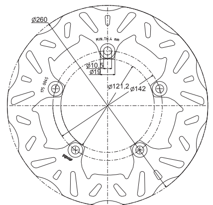
175.0045 thickness/spessore 4,5 mm.
