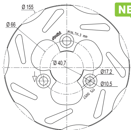
175.0057 thickness/spessore 3 mm.
