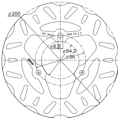
175.0040 thickness/spessore 4 mm.
